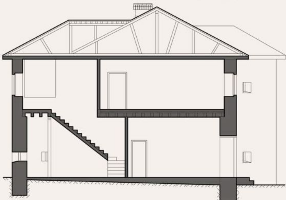
ПОДУЖНИ ПРЕСЕК 1-1
