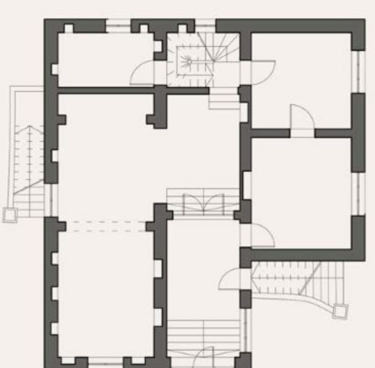
ОСНОВА ПОДРУМА
