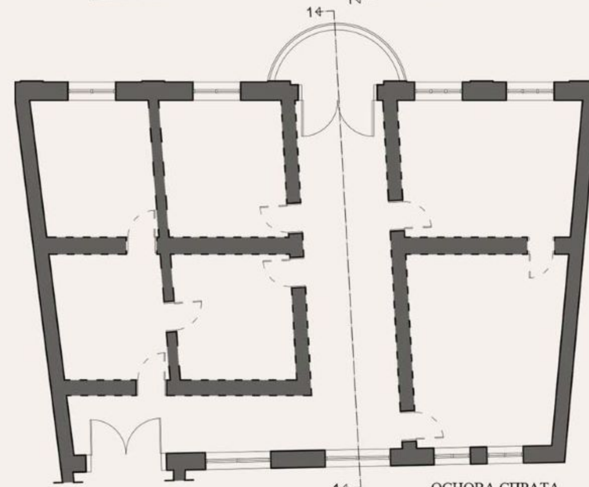
ОСНОВА СПРАТА
