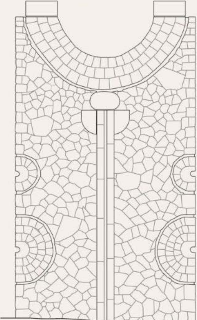
Централна зидана призма (цртеж: ЗЗСК Ниш, Г. Радосављевић, 2016)
