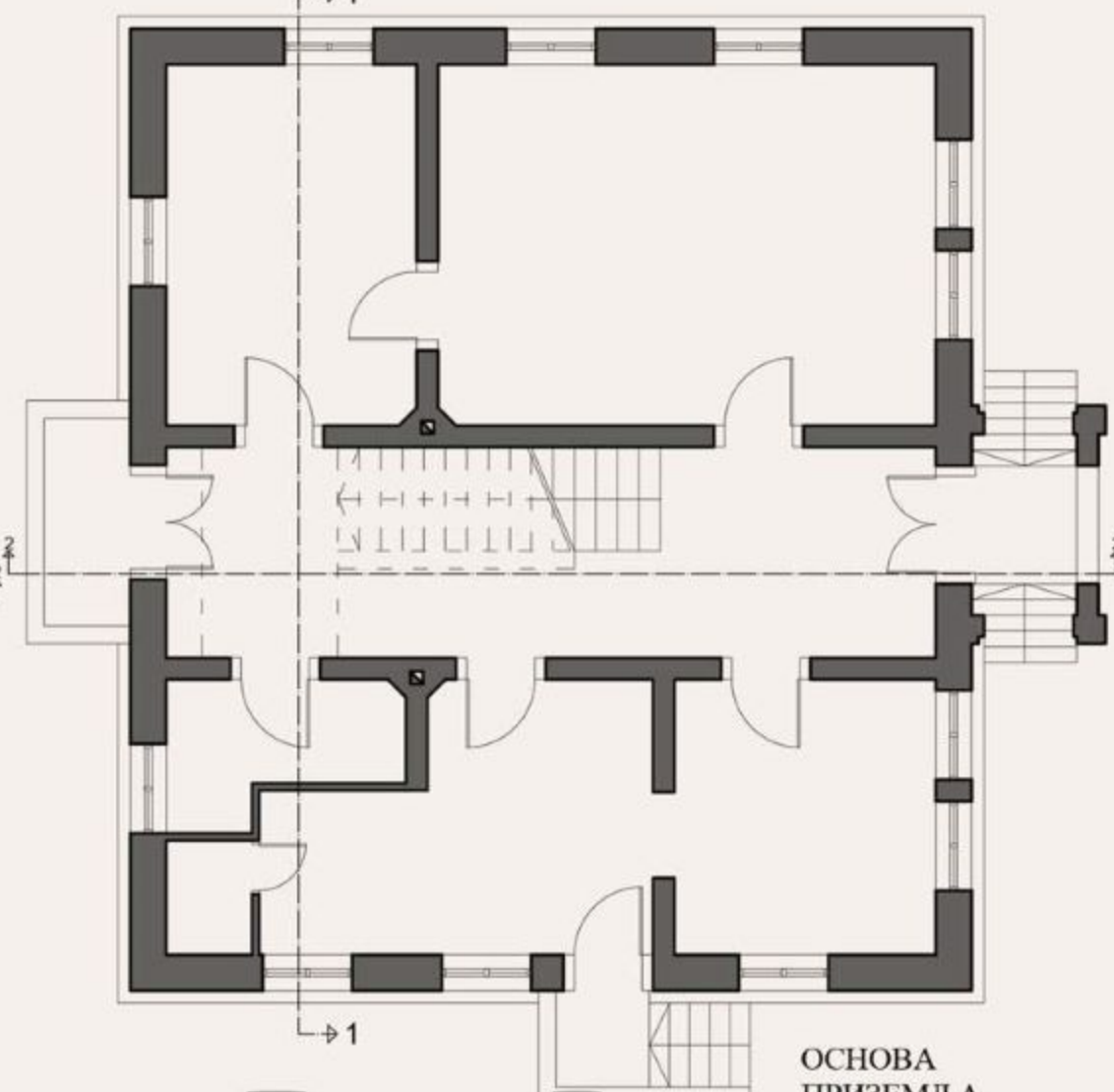
ОСНОВА ПРИЗЕМЉА
