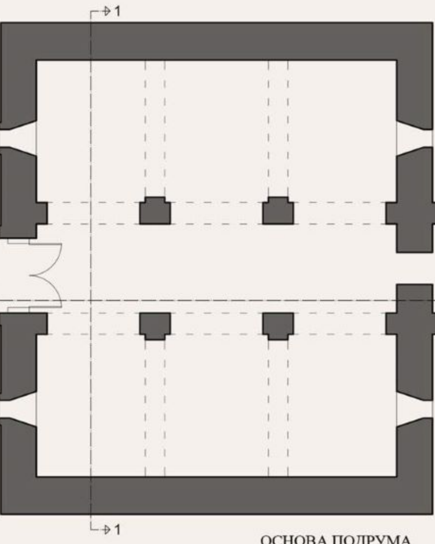
ОСНОВА ПОДРУМА
