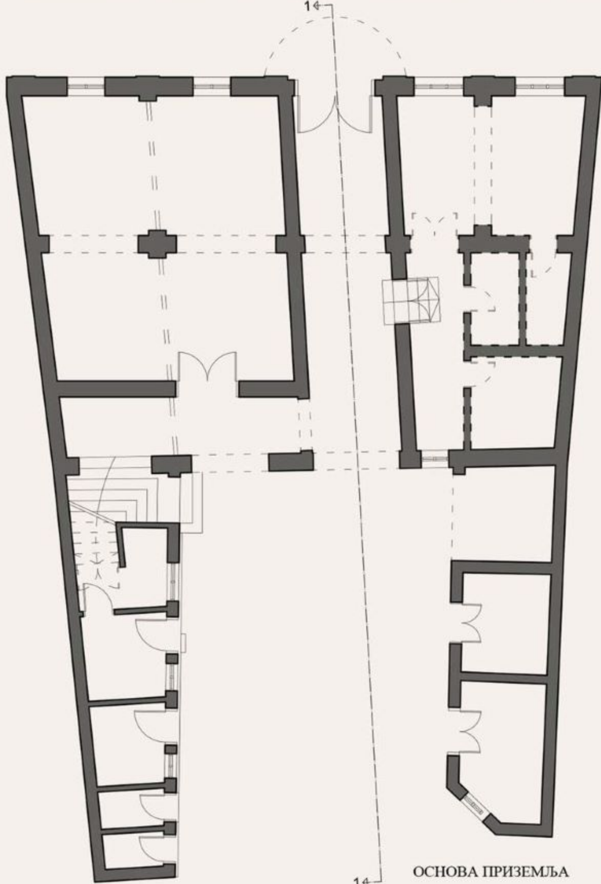
ОСНОВА ПРИЗЕМЉА
