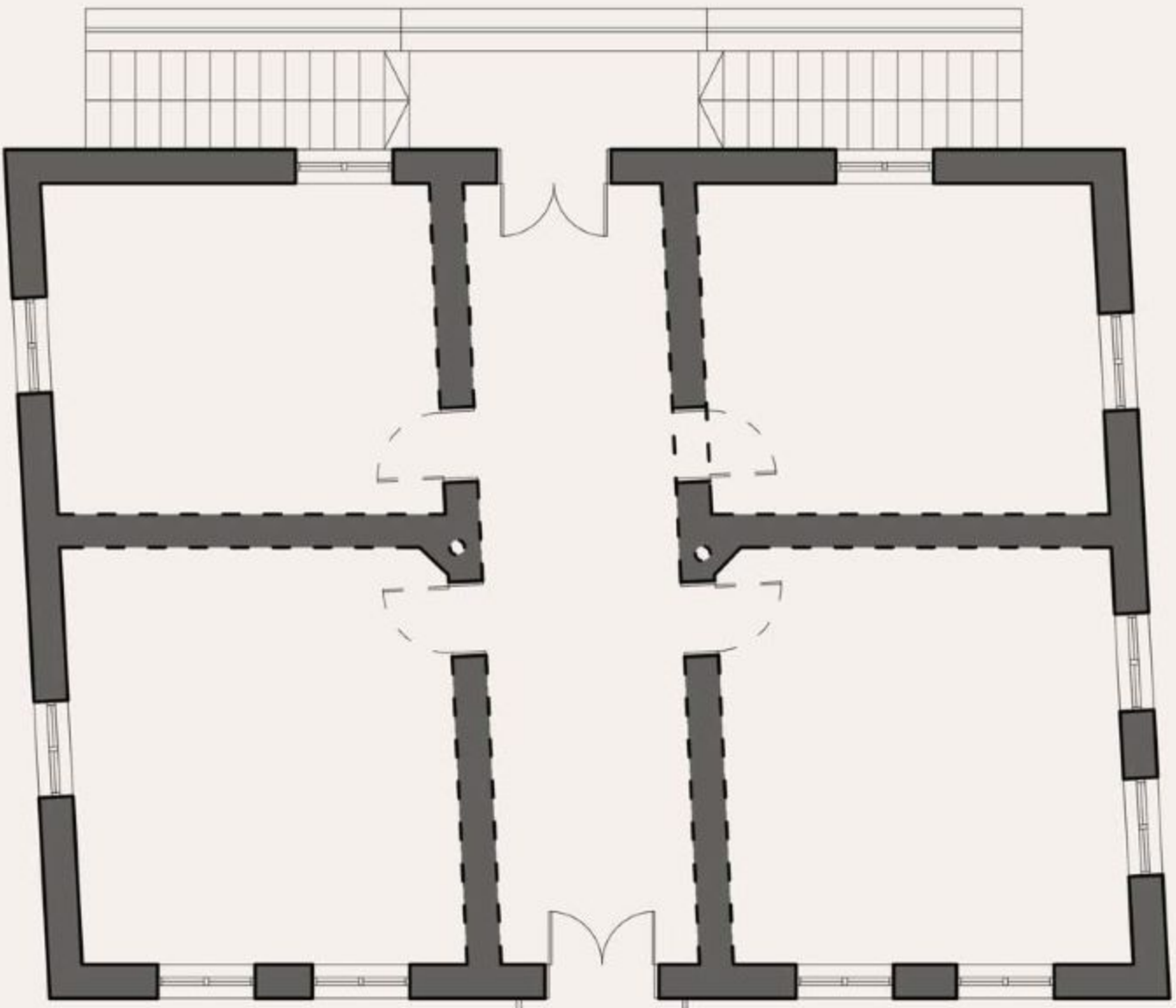
ОСНОВА ПРИЗЕМЉА
