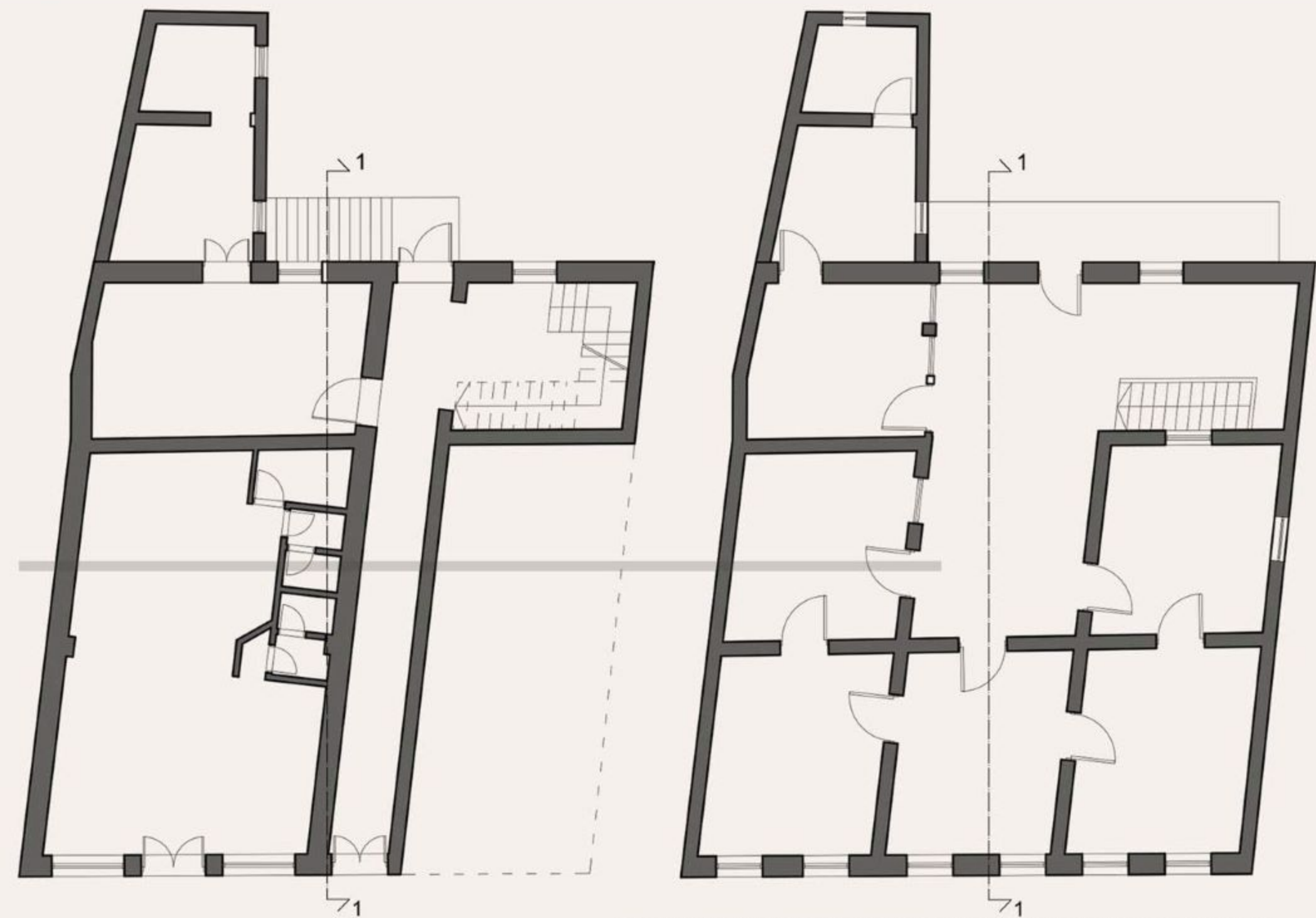
Зграда Илије Краинчанића онова приземља и спрата (цртеж: ЗЗСК Ниш, из приватне архиве власника)
