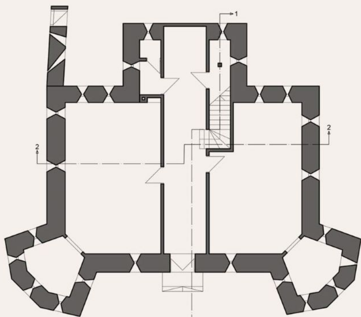
ОСНОВА ПРИЗЕМЉА
