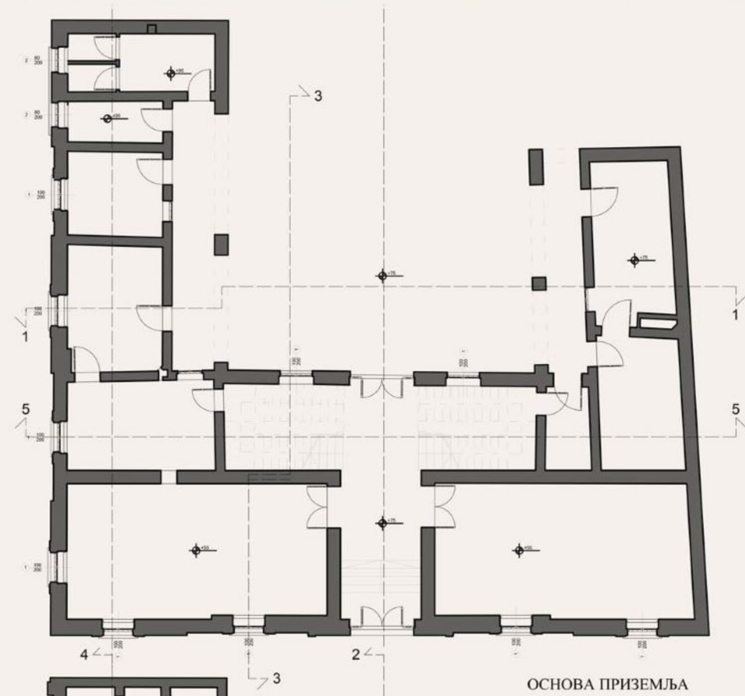
ОСНОВА ПРИЗЕМЉА
