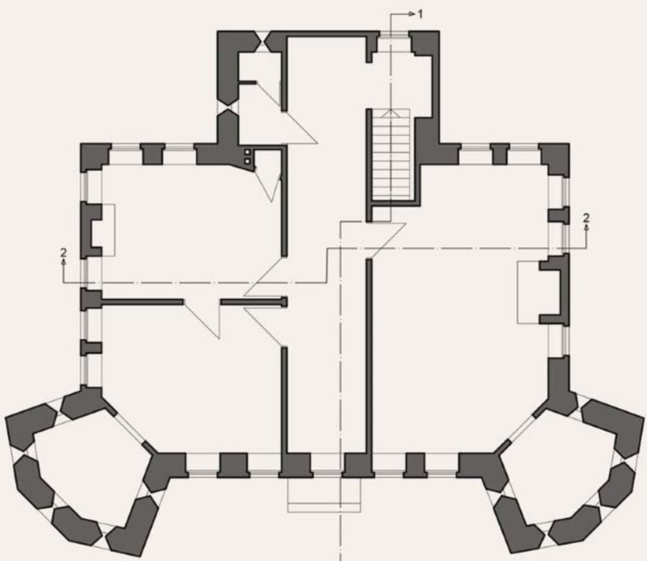
ОСНОВА СПРАТА
