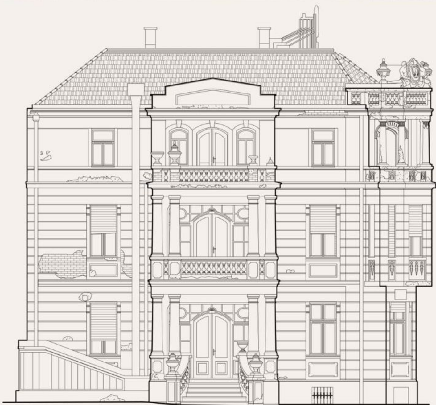
ДВОРИШНА ФАСАДА
