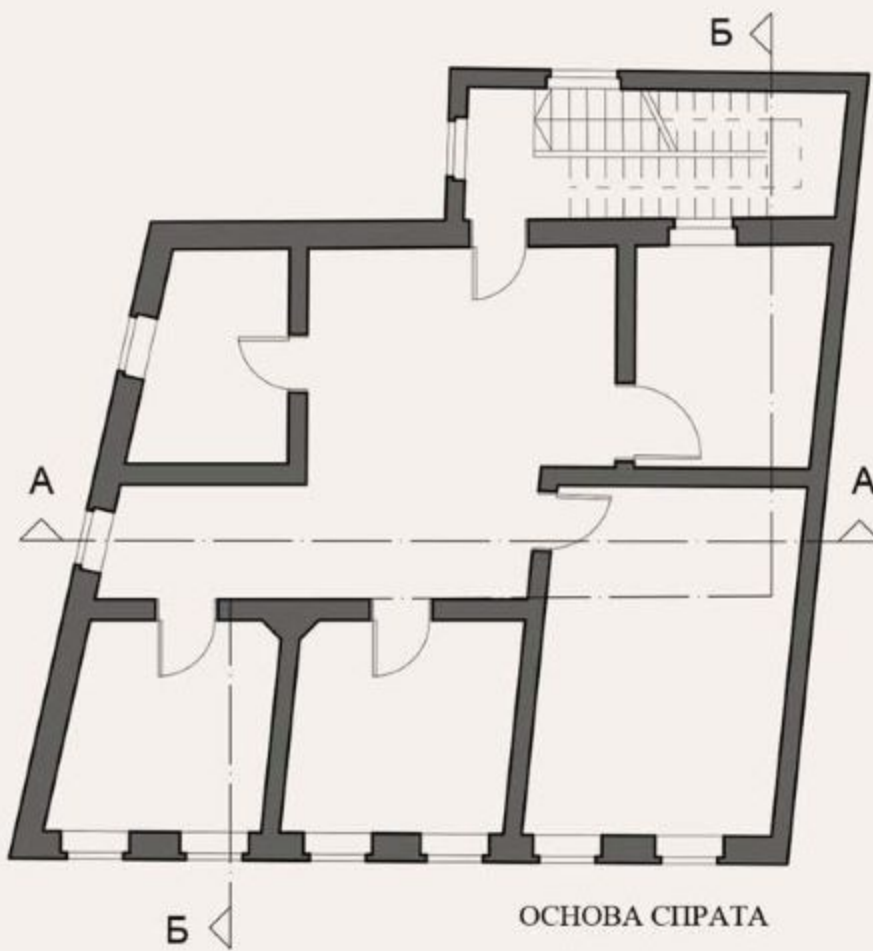
Кућа Ђорђа Поповића (цртежи: ЗЗСК Ниш, на основу архивског пројекта из породичне архиве, обрада: Л. Динић, 2023)
