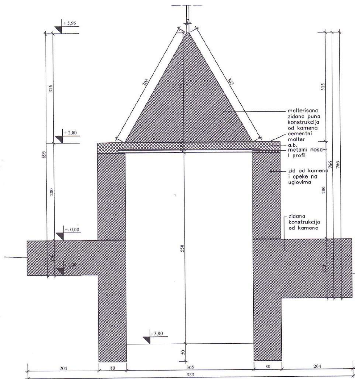
ПРЕСЕК 1-1 Р 1:50
